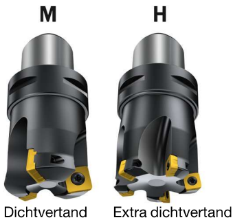
Dichtvertand
